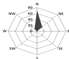
Průměrná četnost směrů větrů (%) za období 25. 2. - 5. 3. 2012
