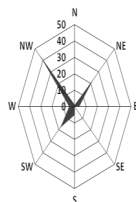
Průměrná četnost směrů větru (%) za období 20. 6. - 12. 9. 2012
